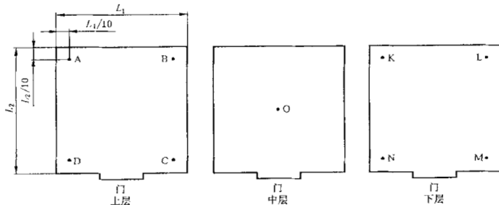
A, B, ..., M, N——温度测试点
